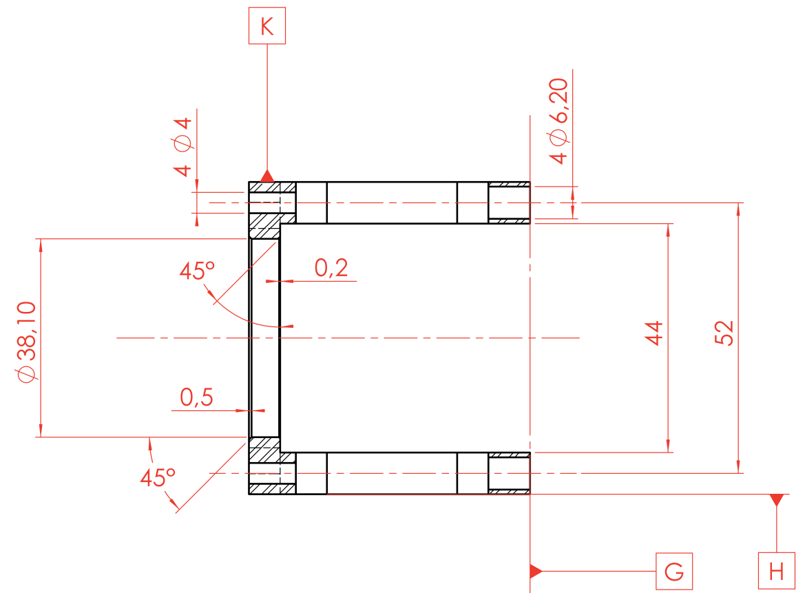
COUPE A-A
